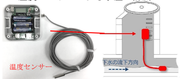
温度センサーによる水温の計測
